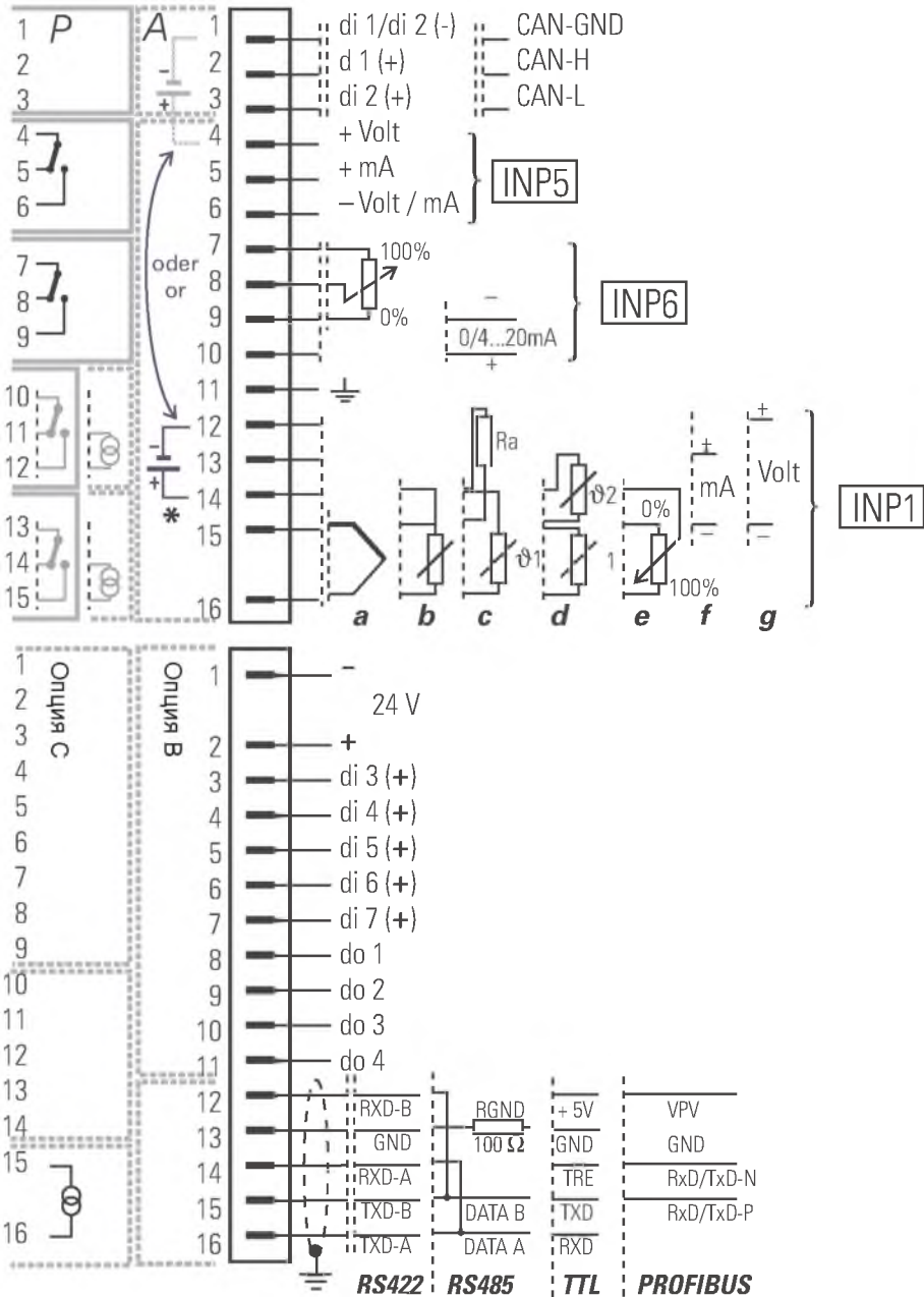
Рис. 12 Электрические подключения
